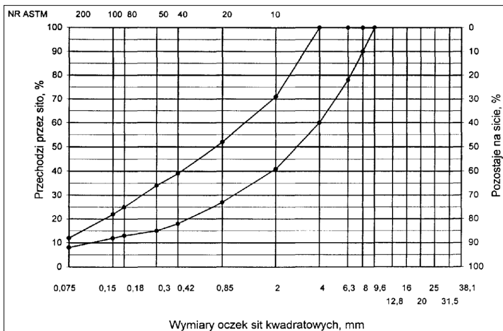
Rys. 3. Krzywe graniczne uziarnienia mieszanki mineralnej BA od 0 do 8mm, od 0 do 6,3 mm do warstwy ścierna nawierzchni drogi o obciążeniu ruchem nawierzchni o obciążeniu ruchem KR1 lub KR2
